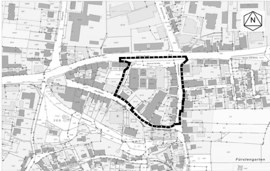
Bebauungsplan Nr. 93 „Östlicher Ortskern“ für den Bereich zwischen Berliner Straße, Fürstengarten, Alte Wache, Am Vorwerk der Stadt Lauenburg/Elbe ■■■■■ Plangrenze
